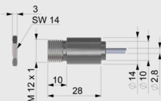
Dimensions optris® CSmicro 3M SF/3M CF
